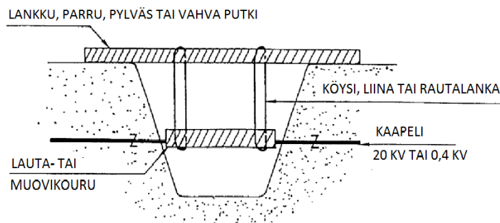
Kaapelien tuenta paikalleen niitä siirtämättä poikittaiskaivannossa
