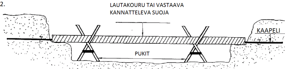
Kaapelien tuenta paikalleen niitä siirtämättä pitkittäiskaivannossa
